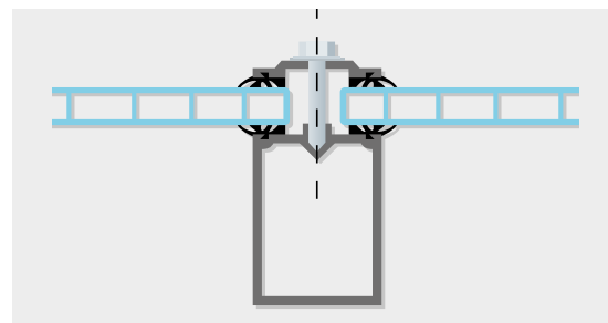
Profilsystem mit voreingestelltem Anpressdruck.
