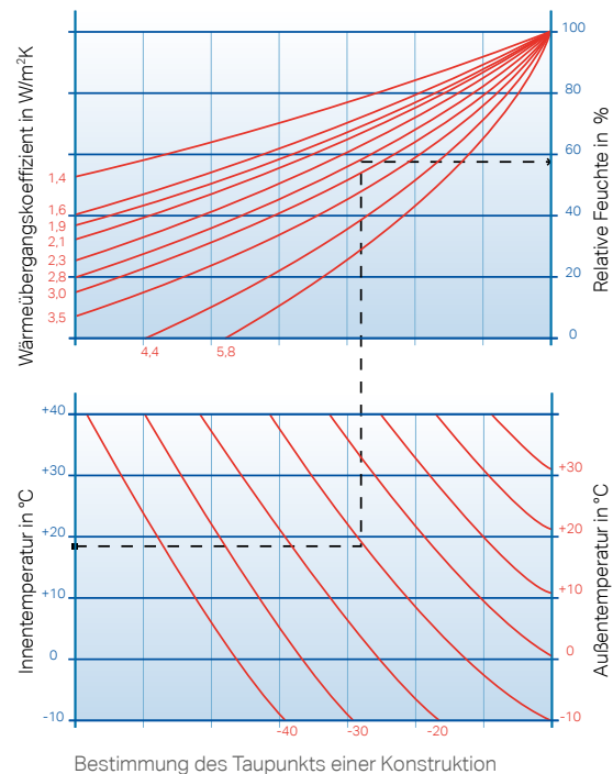
Bestimmung des Taupunkts einer Konstruktion
