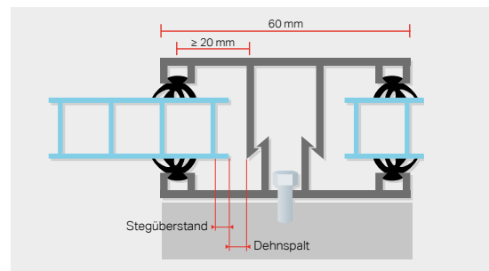
Einspanntiefe
