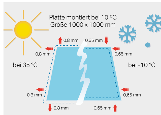
Thermische Ausdehnung
