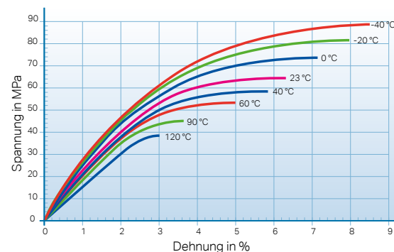
Zugspannung von Exolon® im Verhältnis zur Temperatur.
