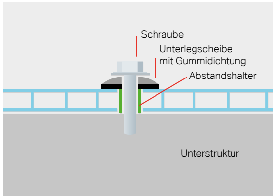
Sogsicherungsschrauben
