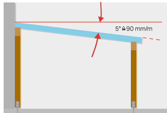
Empfohlener Neigewinkel für Plattenlängen bis zu 6 m.
