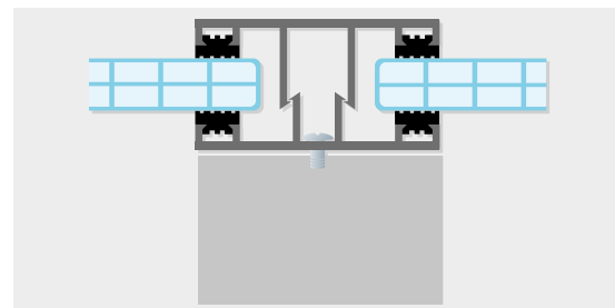
Typische Profilsysteme und Abdichtungen
